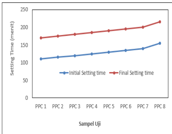
Gambar 4. Pengaruh penambahan fly ash terhadap setting time
