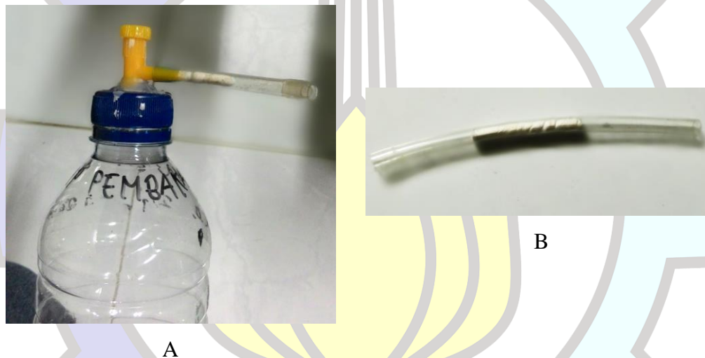
Gambar 3.13 (A) Tempat penyimpanan gas sementara. (B) Selang Berbentuk Tabung Dilengkapi dengan Filter Kertas Tisu
