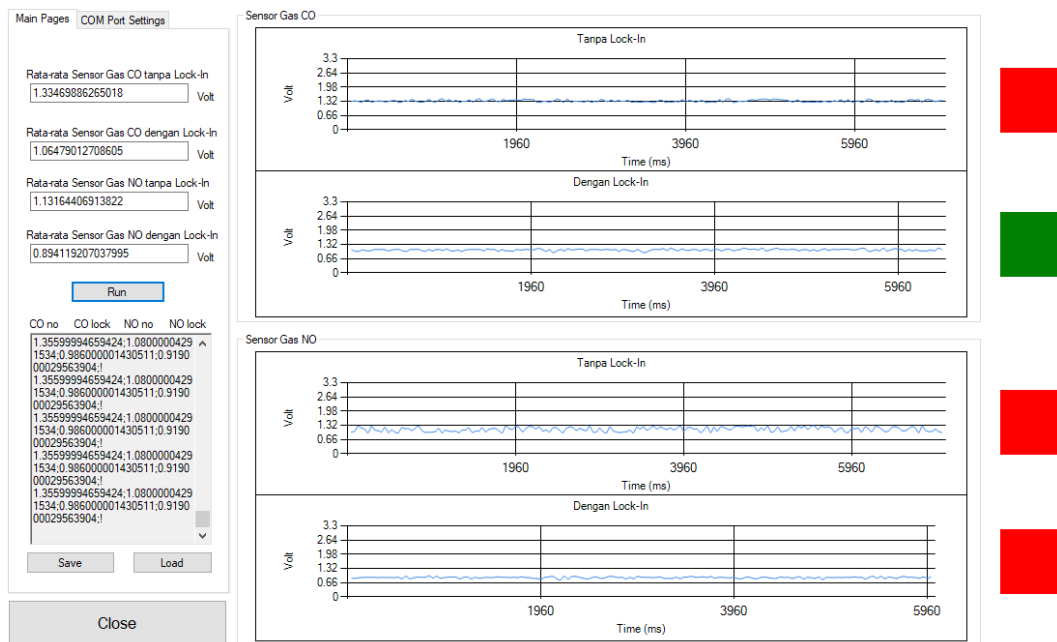
Gambar 4.18 Tampilan GUI pada Rekam Ketiga
