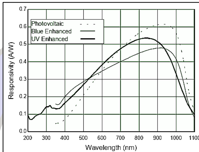
Gambar 3.14 Karakteristik Umum Responsivitas Berbagai Macam Fotodiode Planar Terdifusi Terhadap Panjang Gelombang [31]
