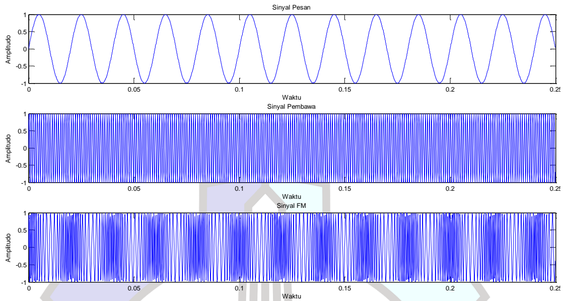
Gambar 4.6 Simulasi Modulasi Frekuensi Sinyal Pesan dengan Sinyal Pembawa Berfrekuensi Lebih Tinggi
