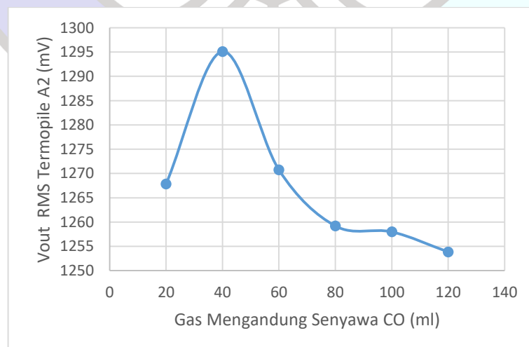
Gambar 4.4 Respon Detektor Termopile A2 Pada Sensor NDIR
