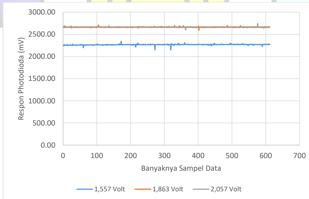
Gambar 4.1 Respon Vout Photodiode Dengan Sumber Daya Lampu Menggunakan Sumber Tegangan ( Voltage Source )
