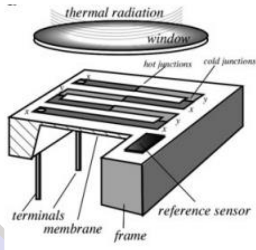
Gambar 2.4 Skematik Detektor Termopile untuk Mengukur Intensitas Sinar Inframerah [16]
